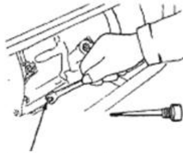
TAMPÃO DE DRENAGEM DO ÓLEO
